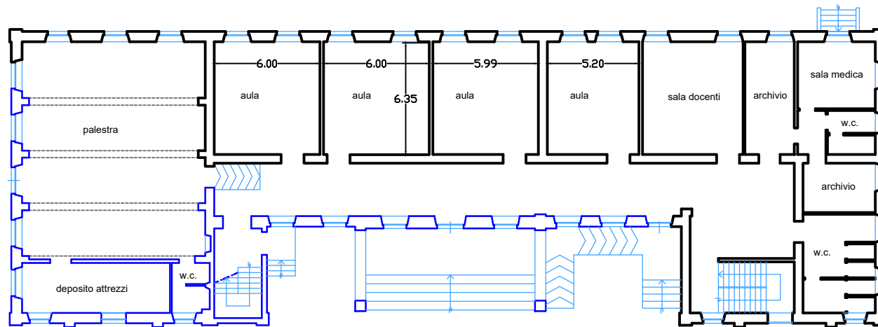
SCUOLA PRIMARIA MORCIANO PIANO TERRA
